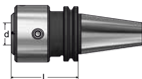
DIN 69871
