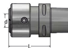
DIN ISO 26623-1
